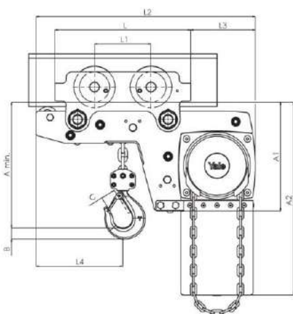
Modèle Yalelift LHP, 500 - 3000 kg, 1 brin
