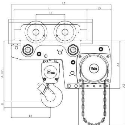
Modèle Yalelift LHP/LHG, 5000 kg, 2 brins
