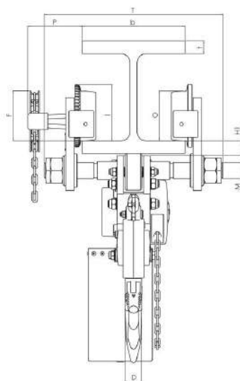
Modèle Yalelift LHG, 500 - 3000 kg, 1 brin
