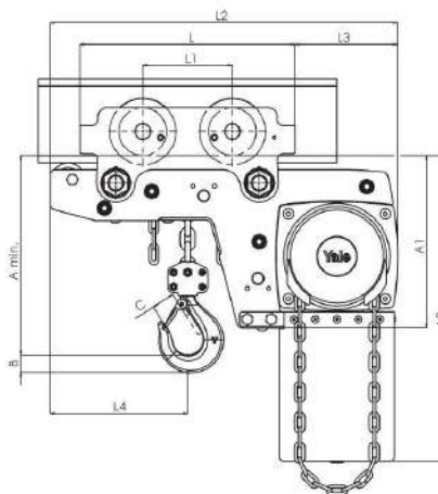
Modèle Yalelift LHG, 500 - 3000 kg, 1 brin
