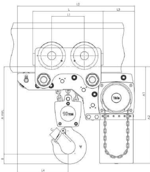
Modèle Yalelift LHG, 10000 kg, 3 brins
